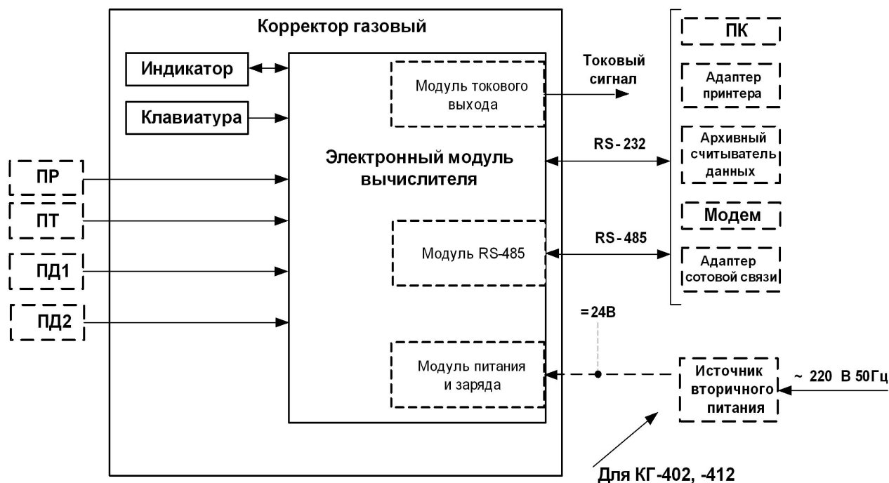
Рис. 1. Структурная схема КГ.
