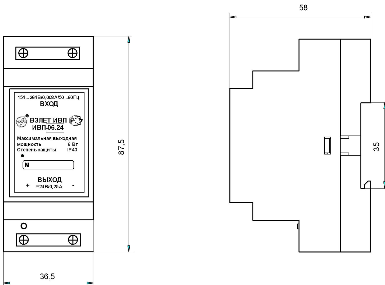
Рис. А.5. Источник вторичного питания «ВЗЛЕТ ИВП» исполнения ИВП-06.24 для электропитания КГ-402, -412
