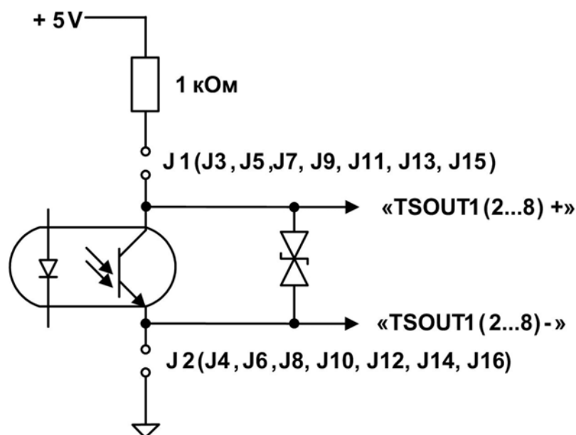
Рис. Б.1. Схема окончного каскада универсальных выходов комплекса
