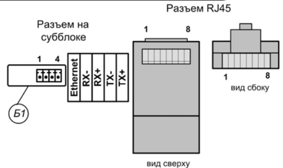
Рис. А.3. Обозначения коммутационных элементов на субблоке вычислителя ТЭР, расположенные на тыльной стороне крышки прибора
