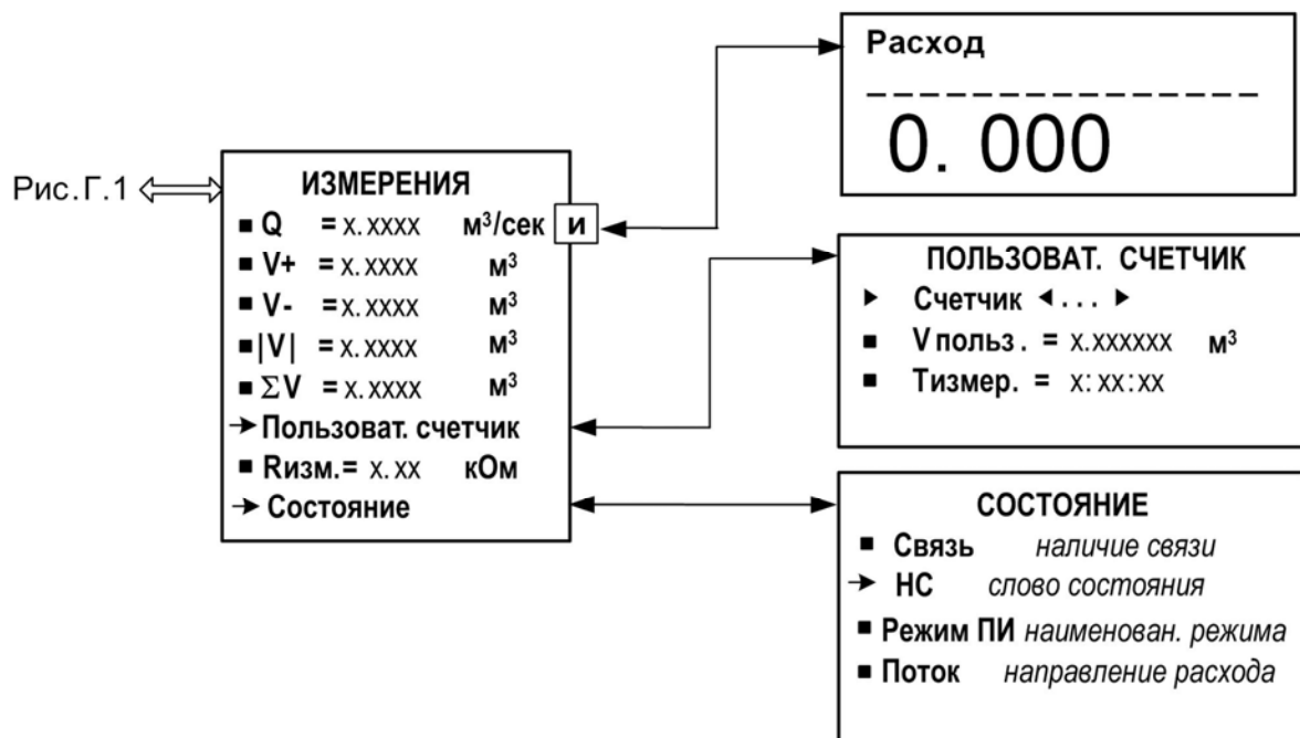
Рис. Г.2. Меню ИЗМЕРЕНИЯ и меню (окна) нижнего уровня
