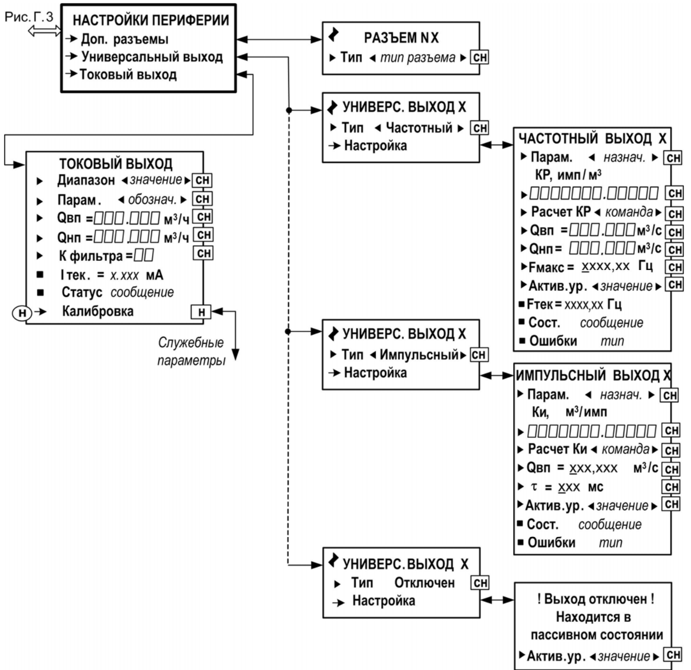
Рис. Г.5. Меню НАСТРОЙКИ ПЕРИФЕРИИ и меню (окна) нижнего уровня
