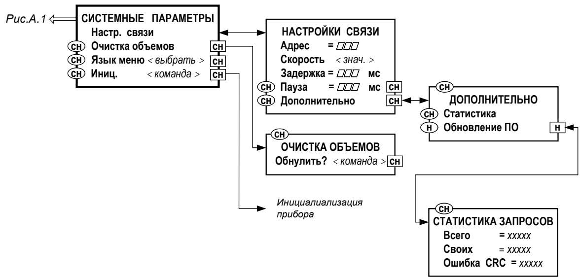
Рис.А.5. Меню «Системные параметры».
