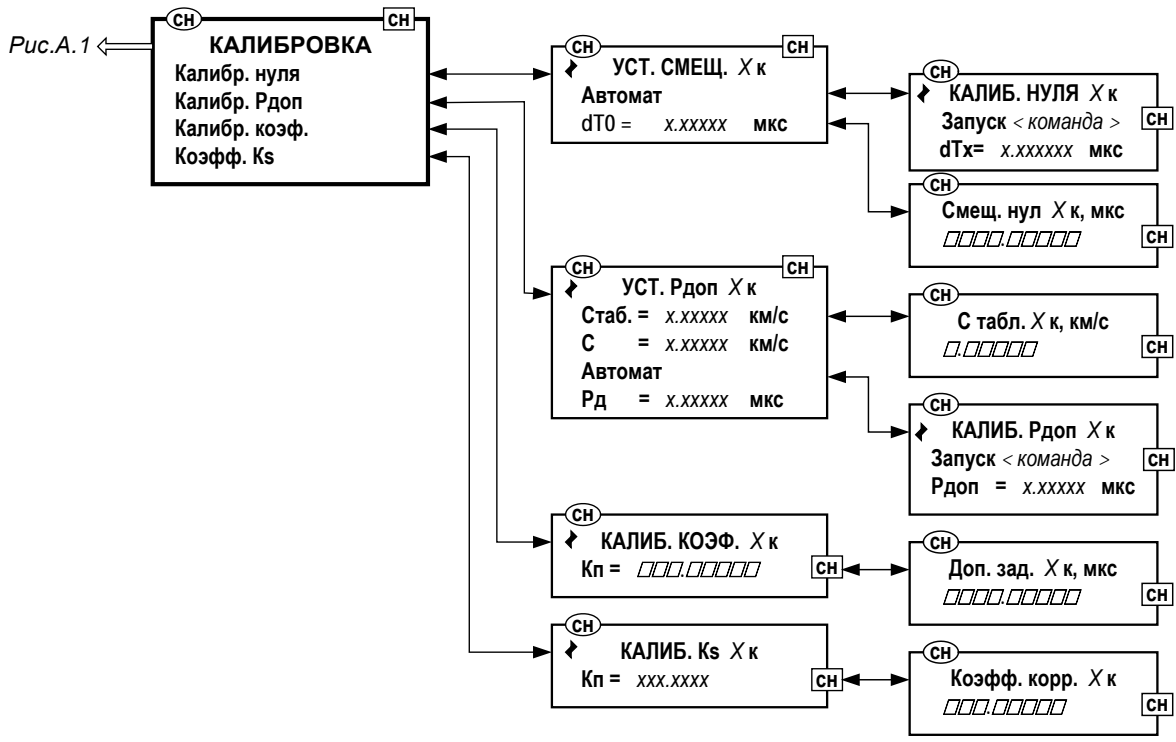
Рис.А.4. Меню «Калибровка».
