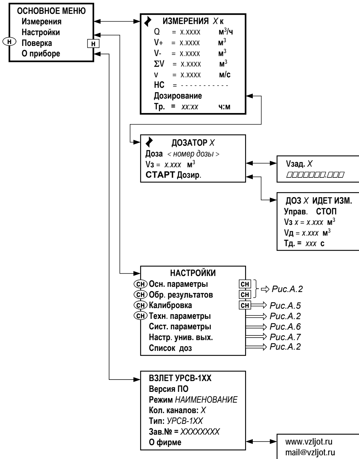
Рис.А.1. Основное меню, меню «ИЗМЕРЕНИЯ» и «О ПРИБОРЕ».
