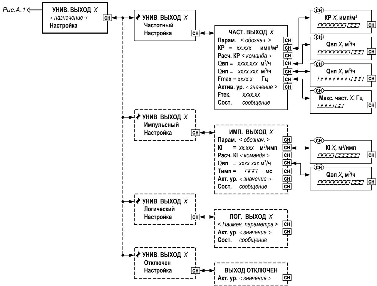
Рис.А.6. Меню настройки универсальных выходов
