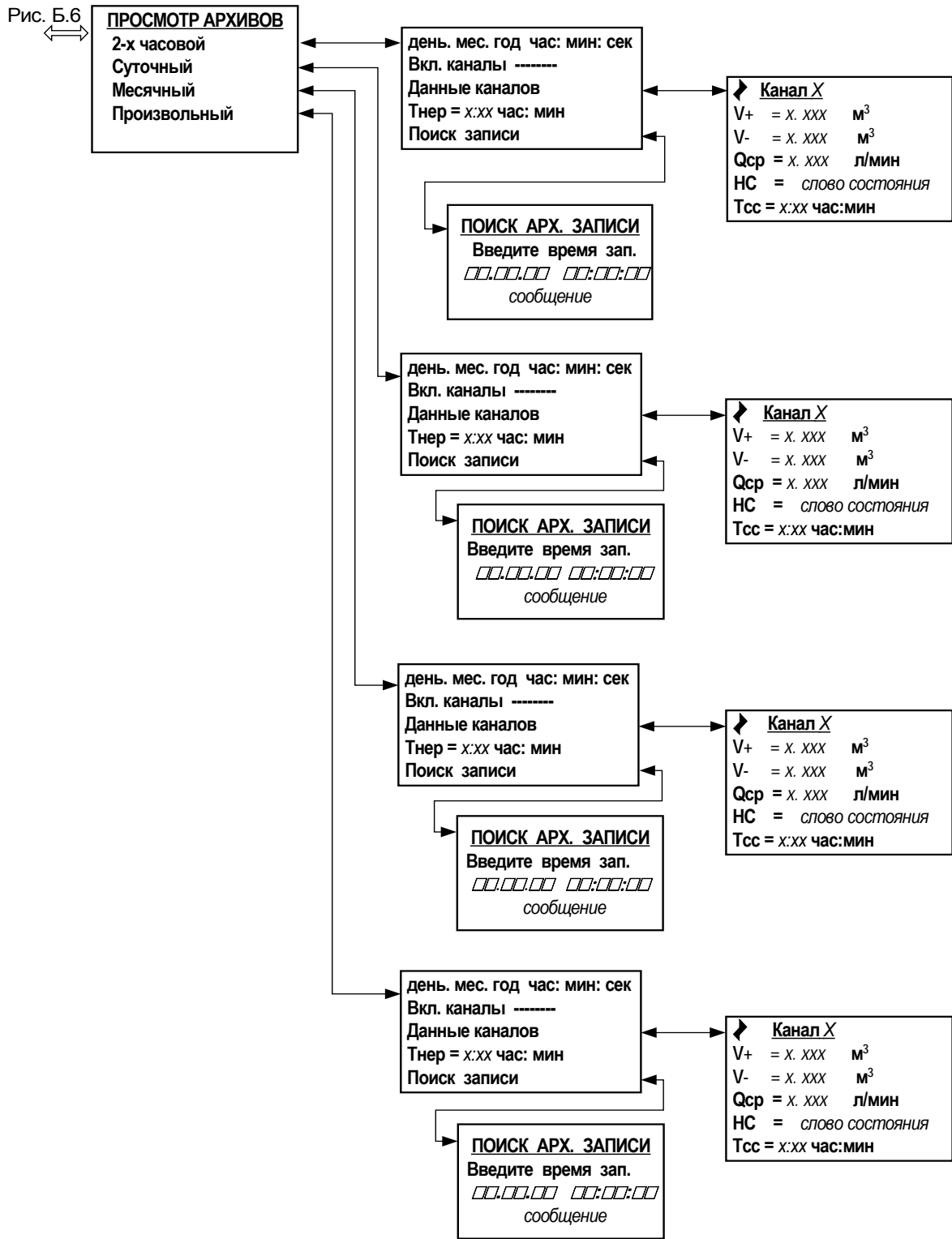
Рис.Б.7. Меню и окна канальных архивов.
