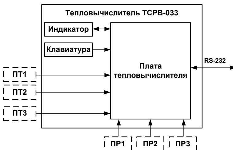
Рис. 1. Структурная схема тепловычислителя исполнения ТСРВ-033.
