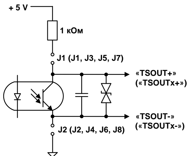
Рис.Ж.1. Схема оконечного каскада универсальных выходов.
