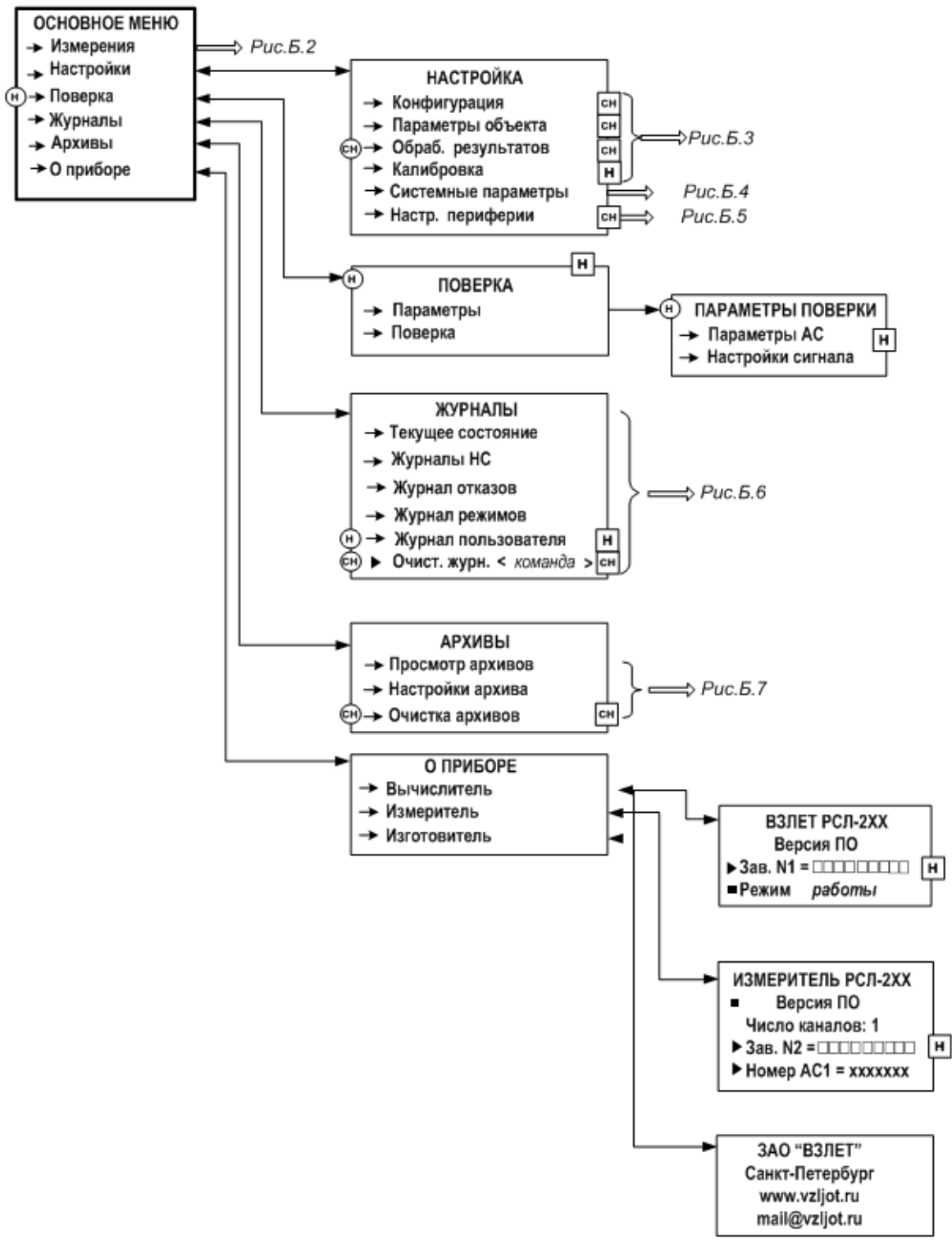
Рис.Б.1. Меню верхнего уровня.
