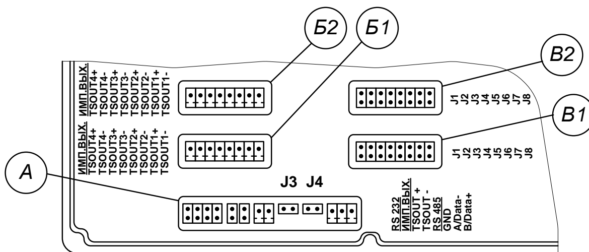
Рис.Е.4. Коммутационные элементы модуля температурных входов.
