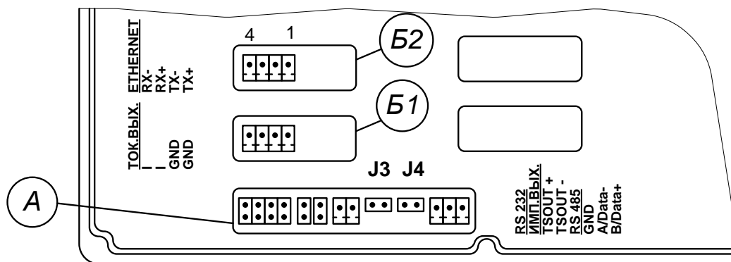
Рис.Е.6. Маркировка коммутационных элементов модулей токового выхода и интерфейса Ethernet.
