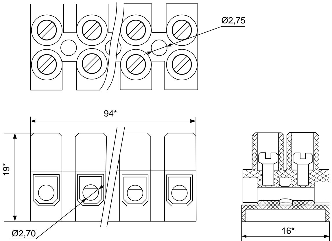
Рис. А.11. Клеммная колодка.
