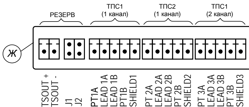
Рис.Е.4. Коммутационные элементы модуля температурных входов.
