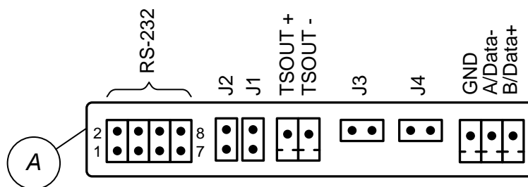
Рис.Е.2. Коммутационные элементы комбинированного модуля.
