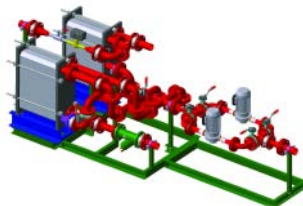
Закрытая система теплоснабжения ГВС через пластинчатый теплообменник
